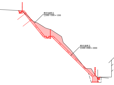
標準断面図
